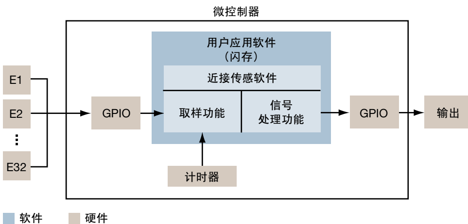
近接传感器软件结构图
