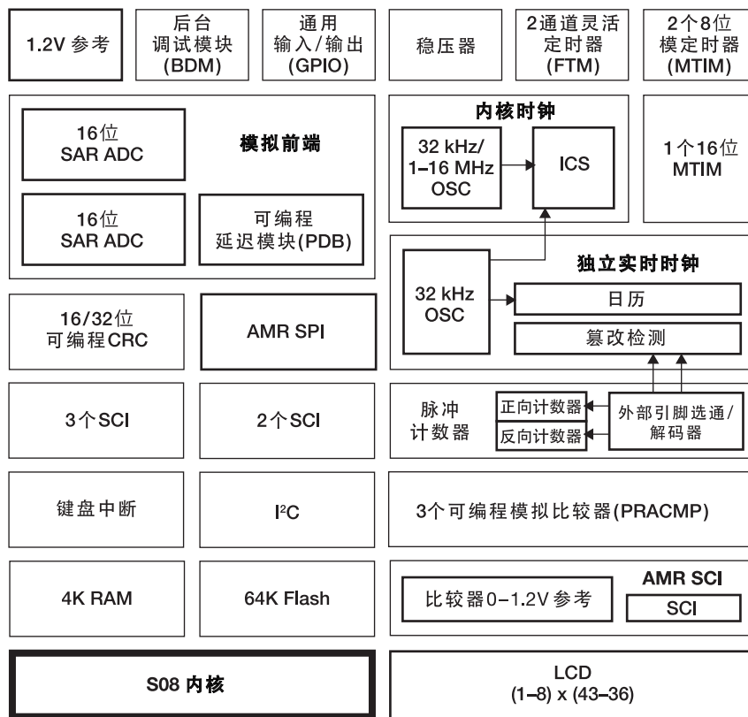
9S08GW 64/32 框图
